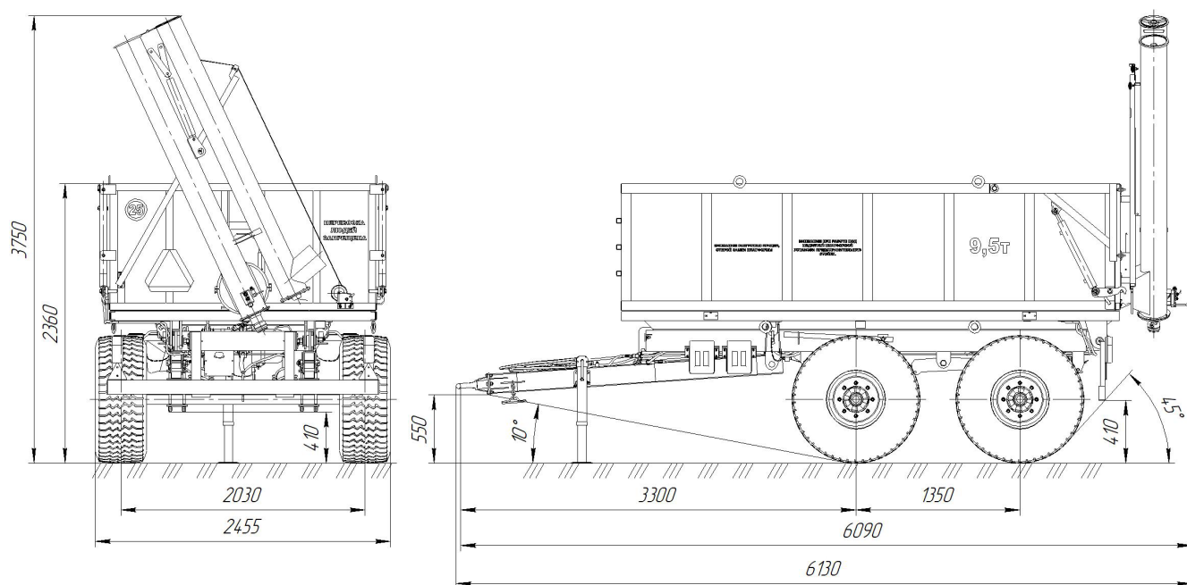
Рисунок 1.3 – Полуприцеп ПТС-9, вариант ПТС-9П
