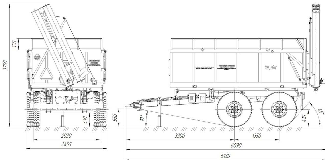
Рисунок 1.4 – Полуприцеп ПТС-9, вариант ПТС-9НП
