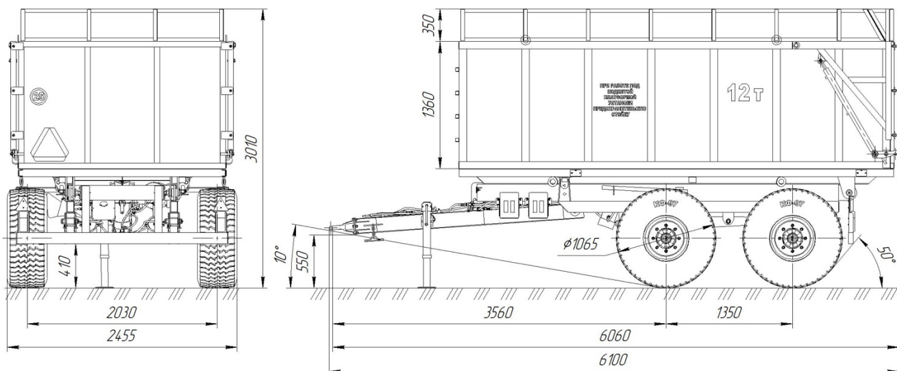
Рисунок 1.2 – Полуприцеп ПТС-12, вариант ПТС-12Н
